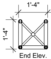
End Elev.
