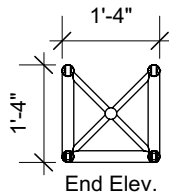
End Elev.
